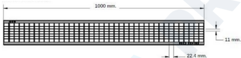
Alzado Lateral
