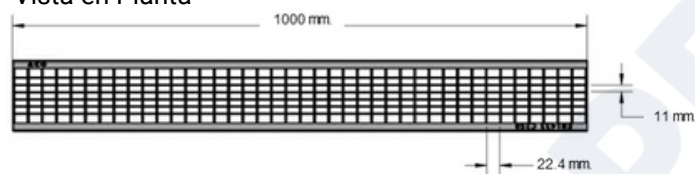
Vista en Planta
