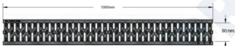
Vista en Planta
