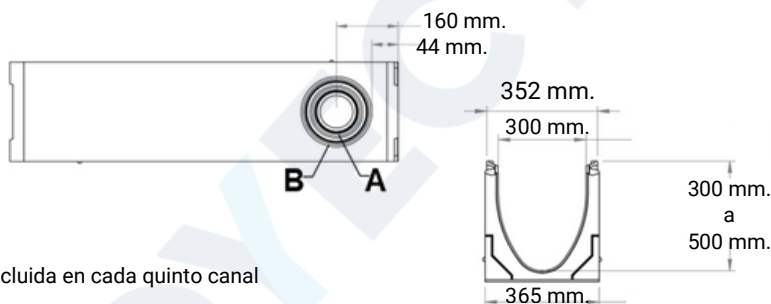
Dimensiones
